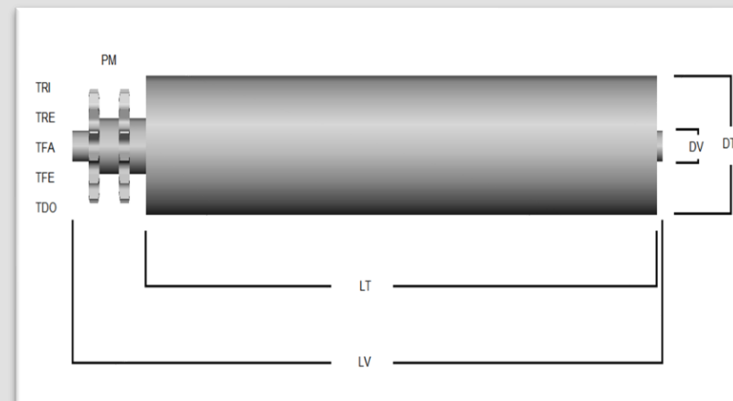
ROLOS MOTORIZADOS / MOTORIZED ROLLS
